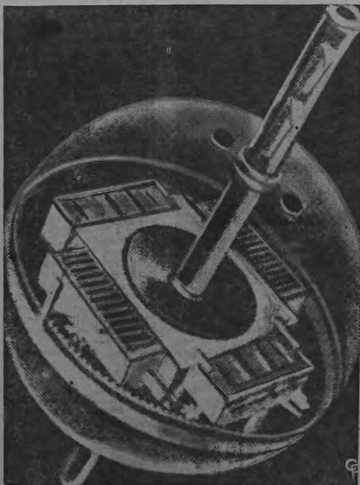
Este dibujo del satélite ruso de la tierra se tomó de una revista soviética. Muestra un corte seccional del interior de la esfera de 184 libras que los rusos llaman "Sputnik" que se puede traducir como "luna artificial".—(INP).
